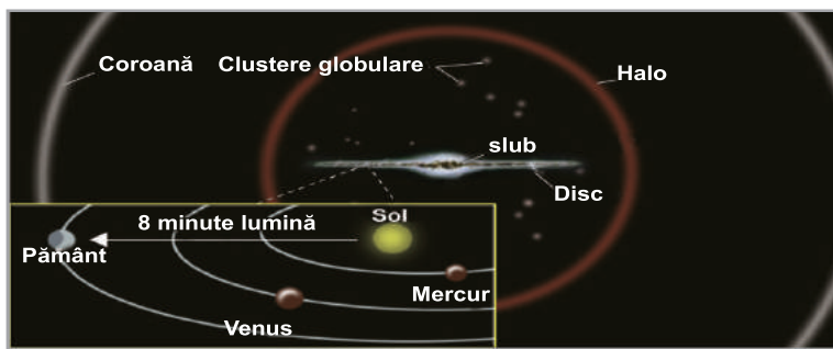
► Această imagine arată expansiunea Universului
