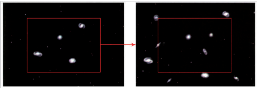
► Figura arată că distanțele dintre Galaxii se află într-o continuă creștere, demonstrând, astfel, că întregul Univers se află în expansiune.
