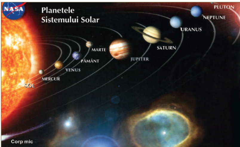
► Galaxia și sistemul solar
