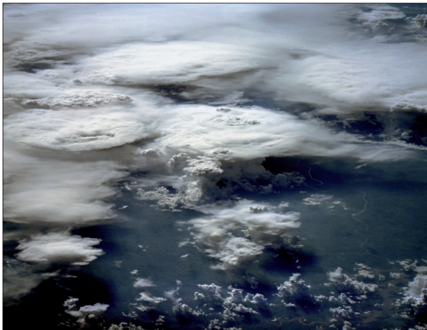
► Un nor cumulonimbus. Imaginea a fost realizată de satelitul NASA. Este ca și cum o mână invizibilă ar împinge norii cumulus spre locul de convergență
