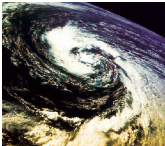
► Imagine a atmosferei, incluzând norii și vânturile
