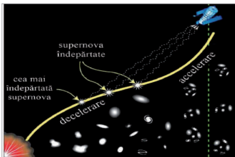
► Figura ilustrează expansiunea Universului
